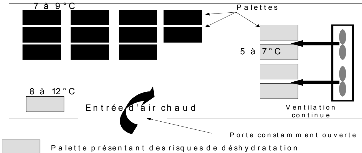
Schéma 3 : Variations des conditions physiques dans une chambre froide - Mesures réelles
